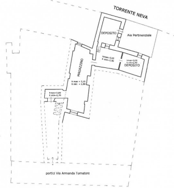
PIANO TERRENO h. scala 3:60
