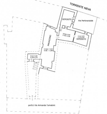
PIANO TERRENO n. scala 2/60
