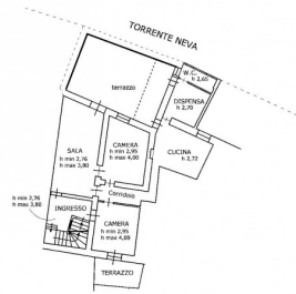
PIANO PRIMO h. scala 2:25
