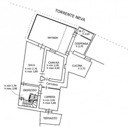
PIANO PRIMO n. scala 2.01
