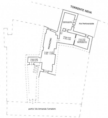
PIANO TERRENO n. scala 3.00
