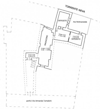
PIANO TERRENO n. scala 2.00
